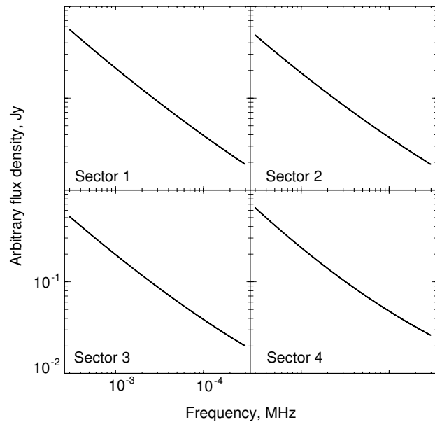
Рис. 5. То же, что на рис. 4, но с осреднением по логарифму плотности потока методом, описанным формулой (2).
